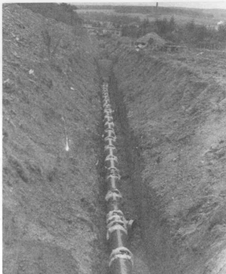
Pohled na čerstvě položený kanalizační řád v novém stavebním obvodu směrem ke Křchlebkám, který je dnes už zahrnut.
